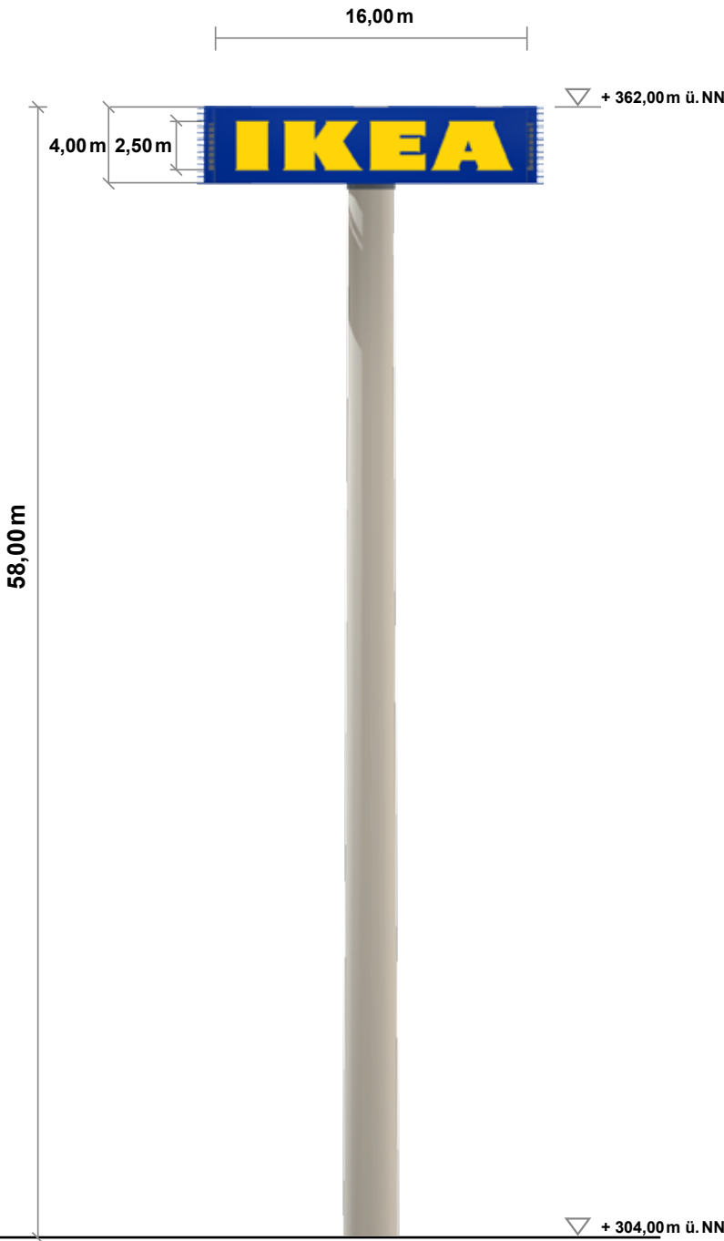
Ansicht Sign-Tower
