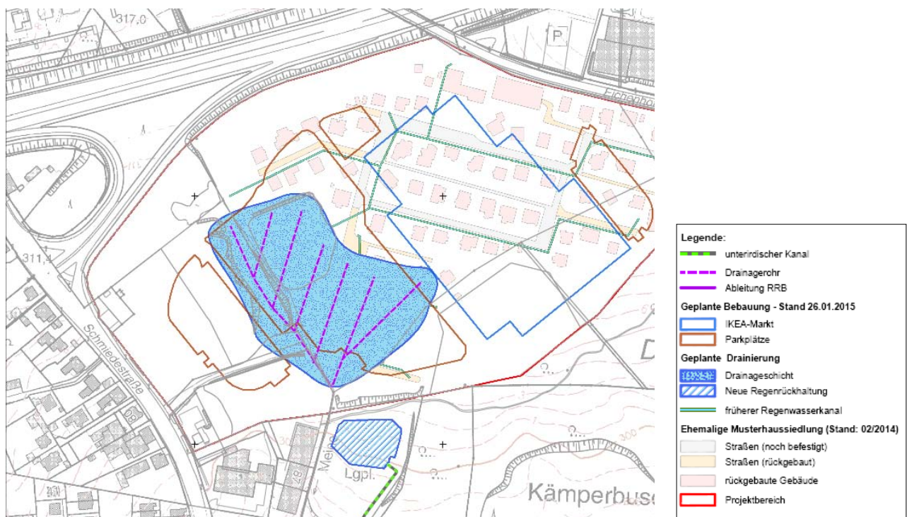
Abb. 11: Lageplan mit Vorschlag zur Drainage des Änderungsbereichs, Quelle: Hydrologisches Gutachten [1].
