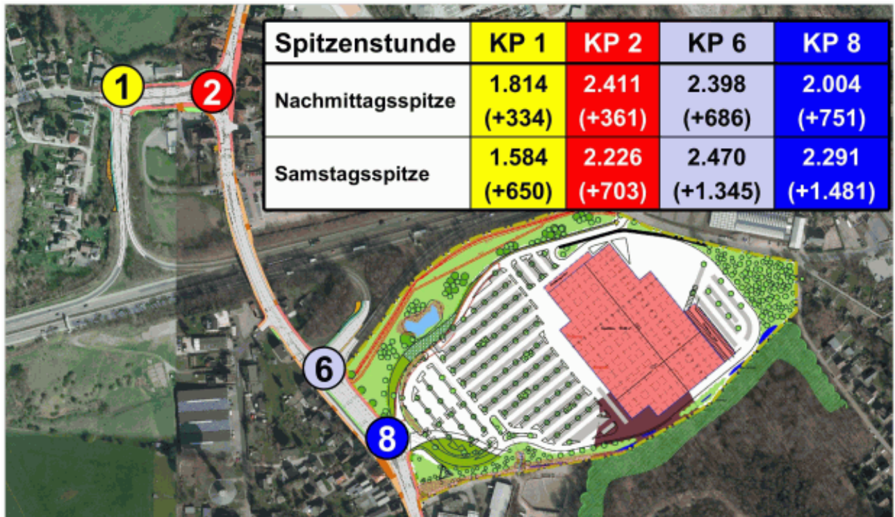
Abbildung 13: Verkehrsbelastungen in den Spitzenstunden (Summe des zuführenden Verkehrs in Kfz/h); Quelle: VUS [9]
