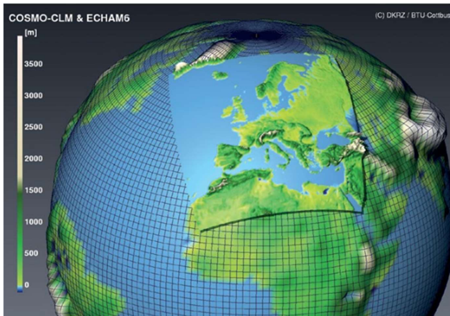
Abbildung 3-2: Beispiel für eine Koppelung eines Globalmodells (hier: ECHAM6) und einem Regionalmodell, hier dem dynamischen regionalen Klimamodell COSMO (CONsortium for Small-scale MOdelling)-CLM bzw. CCLM Modell, das aus dem Wettervorhersagemodell des Deutschen Wetterdienstes entwickelt und durch eine internationale Gemeinschaft von Wissenschaftlern der CLM (Climate Limited-area Modelling)-Community verwendet und weiterentwickelt wird ( http://www.clim-community.eu ). Quelle: DKRZ
