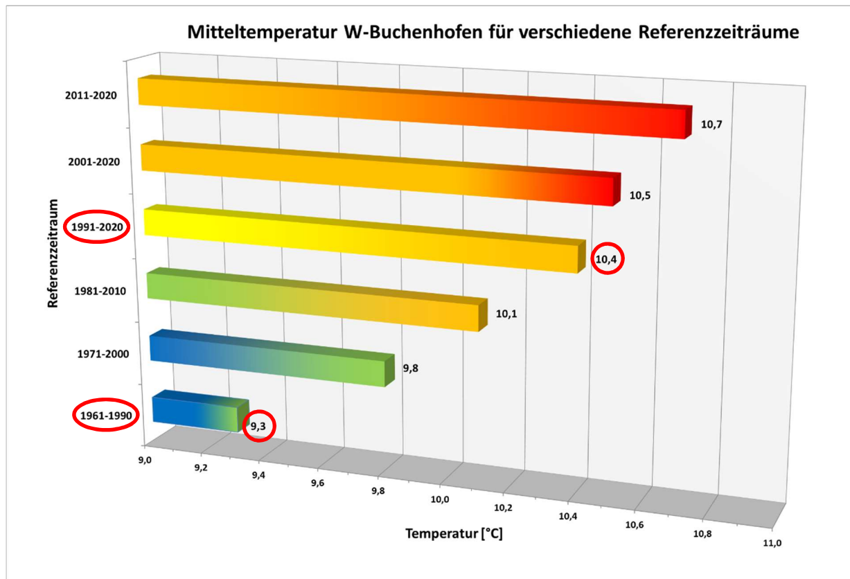
Abbildung 2-15: Mittlere Lufttemperatur verschiedener Zeiträume an der Station W-Buchenhofen. Die „alte“ offizielle Referenzperiode 1961-1990 und die „Neue“ 1991-2020 sind hervorgehoben.
